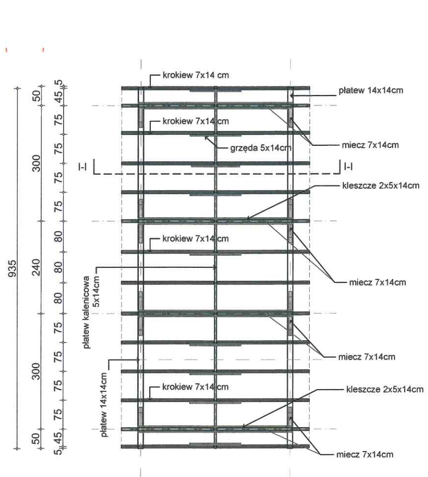
WIĘZBA DACHOWA
