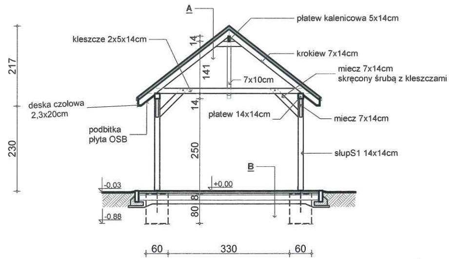
PRZEKRÓJ I-I
