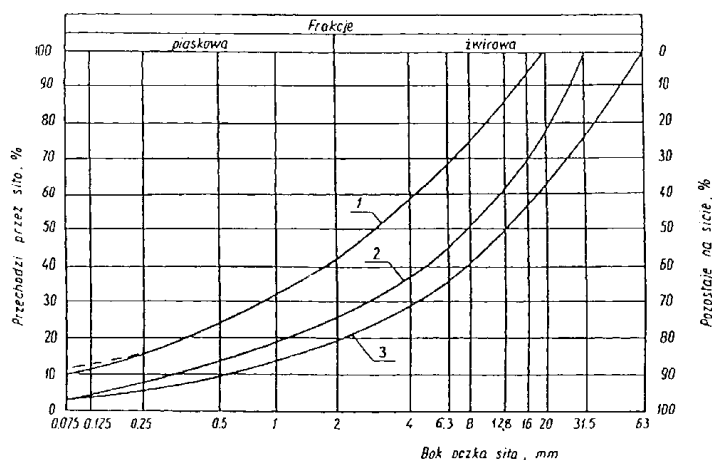
Rysunek 1. Pole dobrego uziarnienia kruszywa przeznaczonych na podbudowy wykonywane metodą stabilizacji mechanicznej 1-2 kruszywo na podbudowę.
